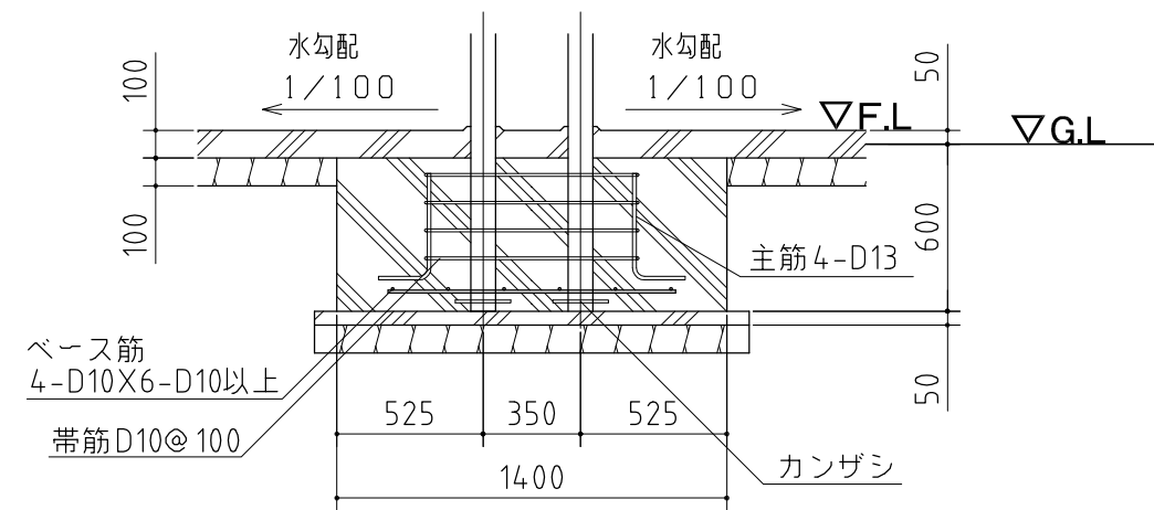
A-A' 断面
